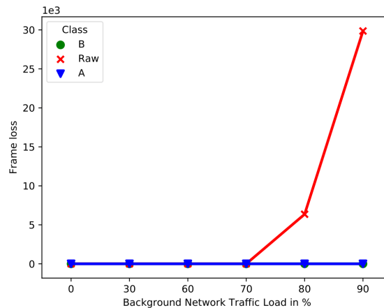
(c) Pérdida de paquetes durante las transmisiones para tráfico de clase A, B y Ethernet (Raw) para distintos porcentajes de tráfico de saturación inyectado.
