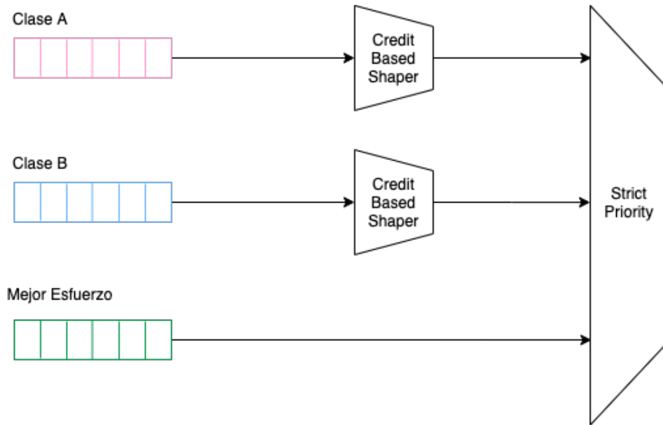
Figura 1.1: Diagrama de las colas de tráfico en un puerto de un switch AVB. CBS trabaja con las colas de clase A y B, mientras que el tráfico de mejor esfuerzo es conformado únicamente por el algoritmo de Strict Priority.
