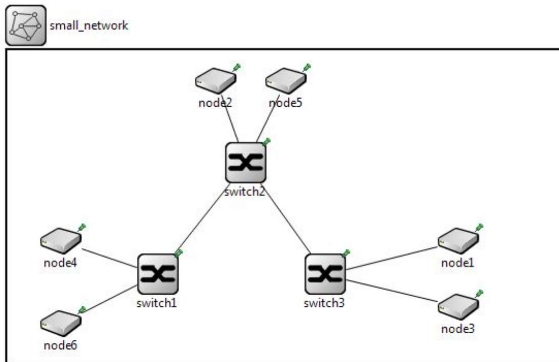
Figura 2.5: Captura de pantalla de la topología Anillo con una conexión menos en simulador OMNeT++. Fue necesario desconectar dos switches para romper con la estructura cíclica, puesto que el framework no la pudo soportar. Una vez realizada la desconexión, la simulación pudo ser completada.
