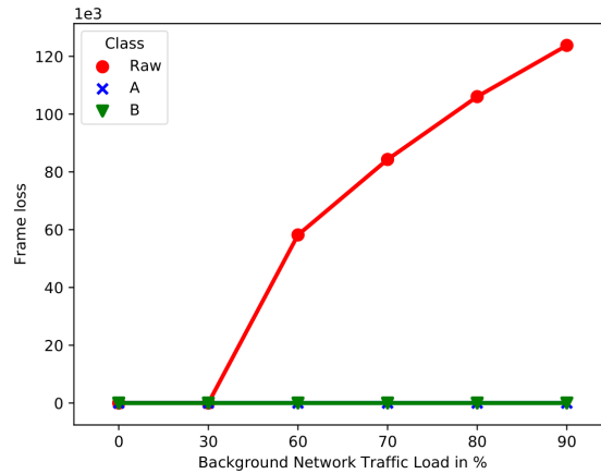
(c) Pérdida de paquetes durante las transmisiones para tráfico de clase A, B y Ethernet (Raw) para distintos porcentajes de tráfico de saturación inyectado.
