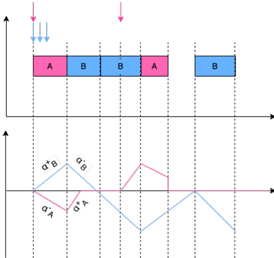
Figura 1.2: Ejemplo de conformado de tráfico realizado por CBS. Mientras una trama es transmitida su cantidad de créditos disminuye según su pendiente de envío ( \alpha^- ) y mientras aguarda a ser transmitida crece según su pendiente de inactividad ( \alpha^+ ). Una trama es transmitida si posee una cantidad positiva de créditos y si no hay una trama de mayor prioridad pendiente.
