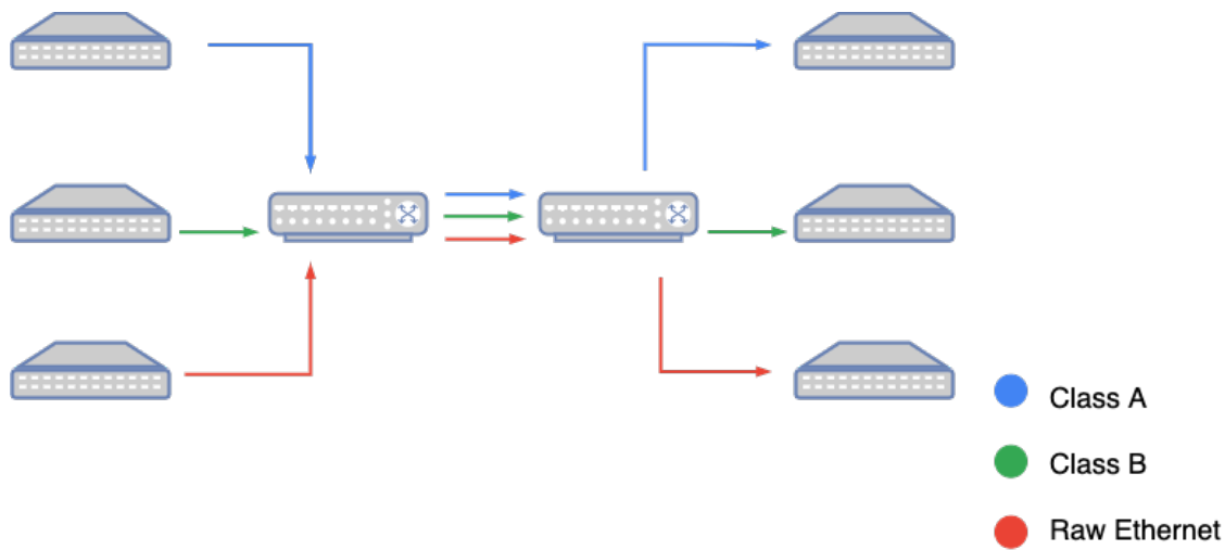
Figura 3.11: Topología realizada para validar el método escogido para obtener el tiempo de encolado dentro del switch. El puerto conectado al segundo switch, de esta manera, es el punto de mayor aglomeración de la red. Se conectan tres dispositivos a cada switch para poder transmitir tres tipos de tráfico: clase A, clase B y mejor esfuerzo.
