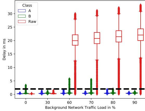
(a) Diagrama de caja para la topología Cadena. En este diagrama se presenta la demora de un extremo a otro para cada tipo de tráfico. La línea punteada negra refleja la demora máxima asegurada por AVB/TSN para tráfico de clase A.
