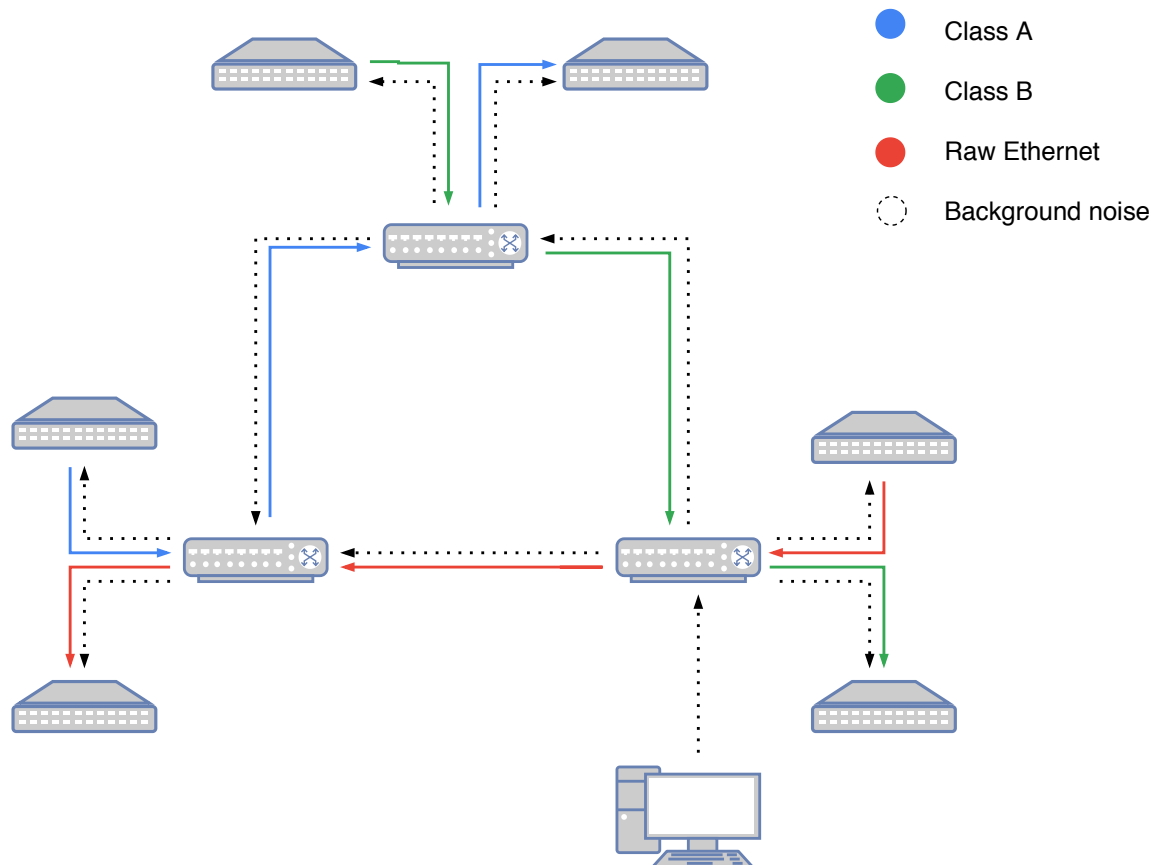
Figura 3.5: Topología Anillo. En esta configuración se conectan los tres switches entre ellos y además se le agregan dos dispositivos a cada uno. Las conexiones se hicieron tales que el tráfico tuviera que fluir por dos switches para llegar a destino. El interés principal de esta topología consiste en su estructura cíclica.
