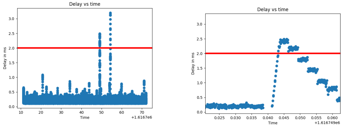
(a) Diagrama de demora vs tiempo de una transmisión de tráfico clase A en la topología Estrella con 85 % de tráfico de saturación.
