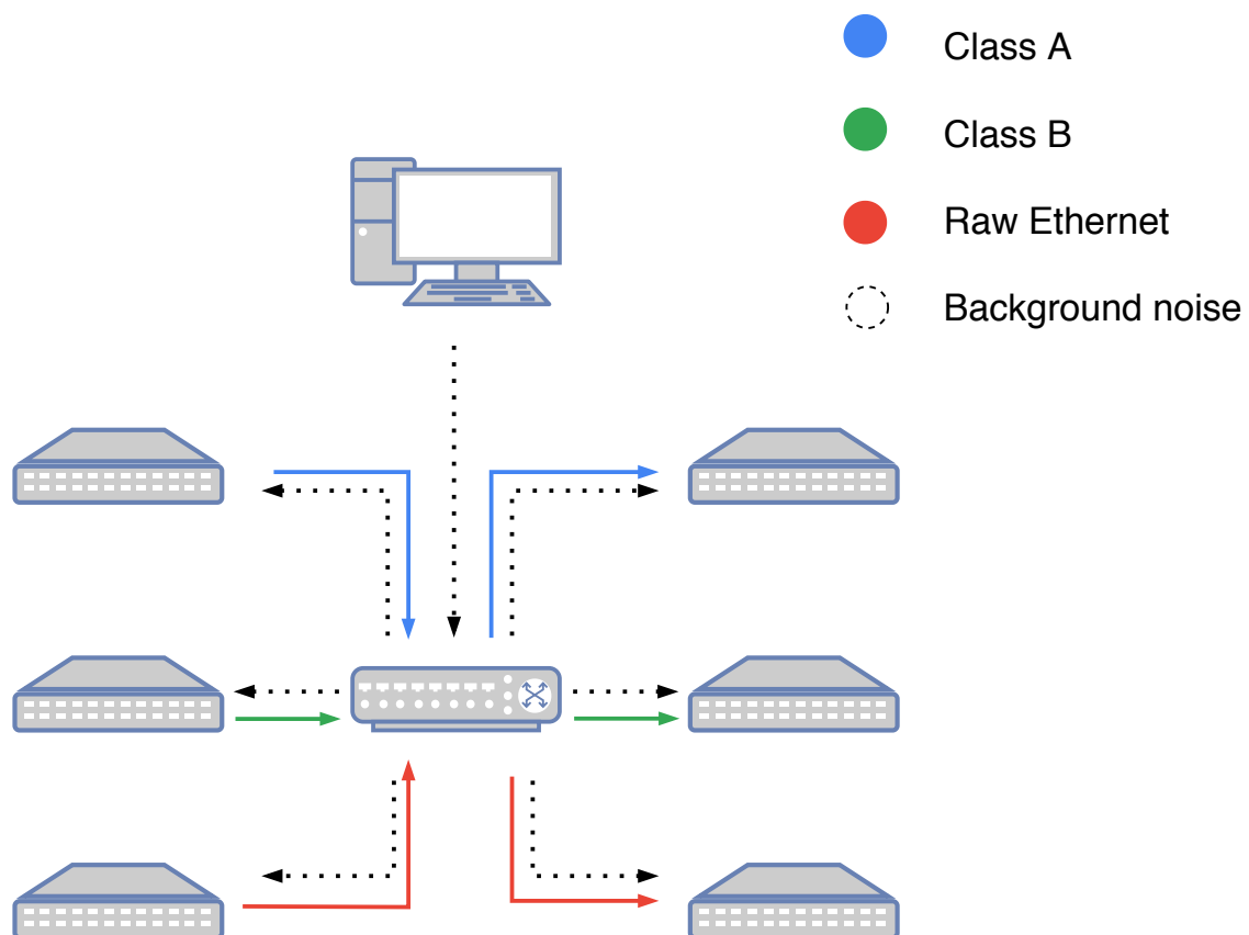
Figura 3.3: Topología Estrella. Esta disposición consiste de seis dispositivos conectados a un switch central. El desafío principal es la generación de un punto de congestión por donde todo el tráfico tiene que viajar.
