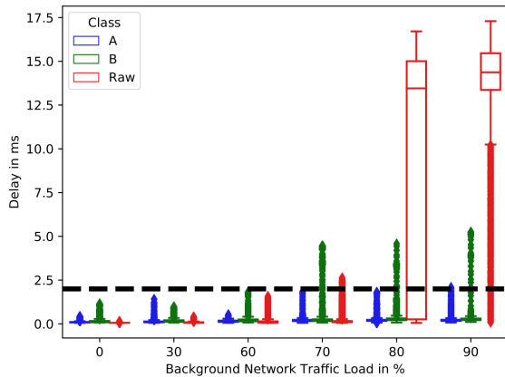
(a) Diagrama de caja. En este diagrama se presenta la demora de un extremo a otro para cada tipo de tráfico. La línea punteada negra refleja la demora máxima asegurada por AVB/TSN para tráfico de clase A.
