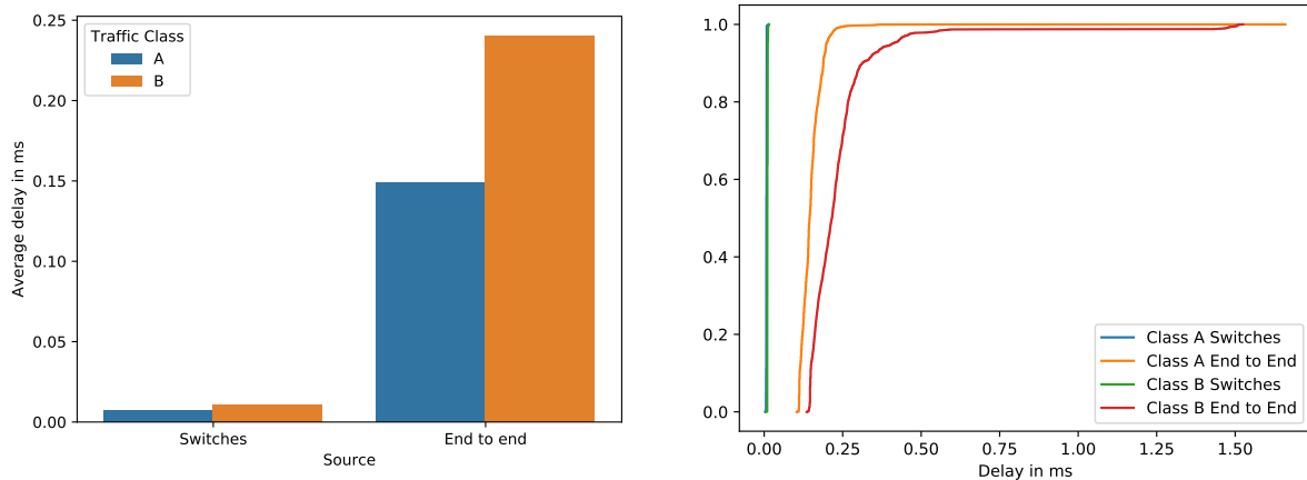
(a) Demora promedio de una trama dentro del switch comparada con la demora de un extremo a otro.
