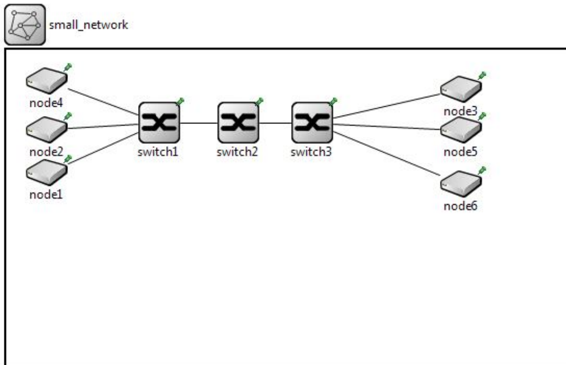
Figura 2.3: Captura de pantalla de la topología Cadena en simulador OMNeT++. Este caso introduce dos switches más en el entorno virtual, lo que permite explorar la conexión de switches entre ellos y el desempeño del protocolo al agregar más puntos de congestión.
