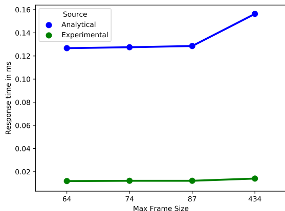
(a) Tiempo de respuesta en milisegundos de tráfico de clase B. En las cuatro transmisiones distintas se varía el tamaño máximo de trama para el tráfico de clase A que se transmite en simultáneo.
