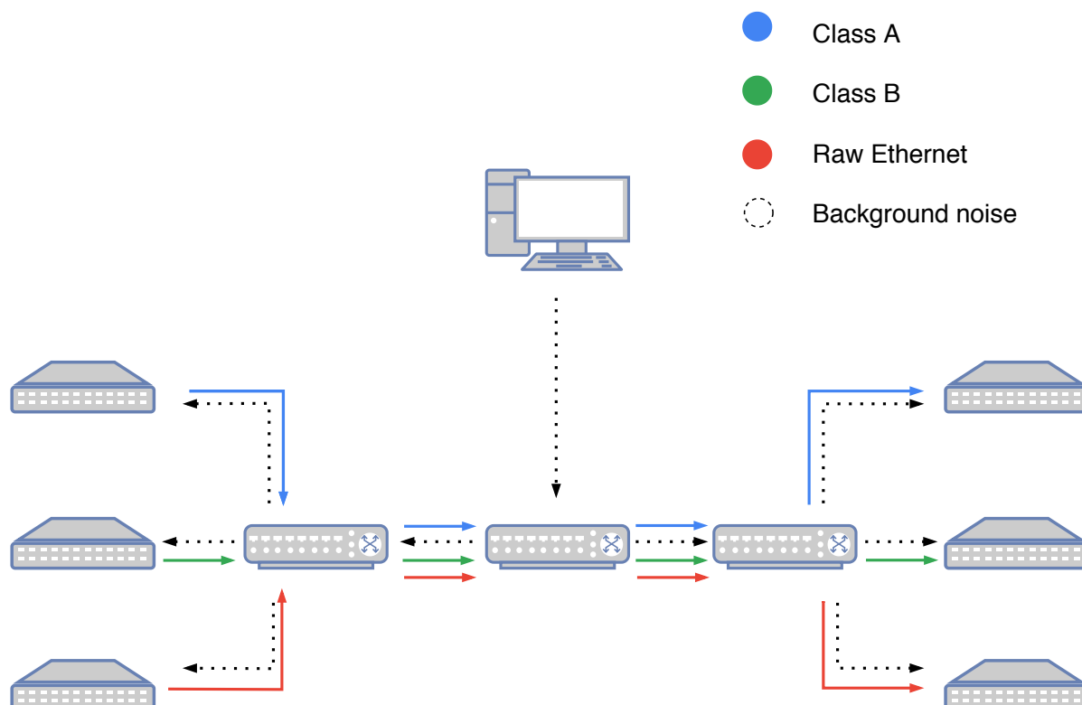
Figura 3.4: Topología Cadena. Esta disposición consiste de seis dispositivos y tres switches. Se agregan dos saltos más por donde debe fluir el tráfico. Además, el switch ubicado en el medio crea un punto de congestión en donde los tres tipos de tráfico sumado al tráfico de saturación de la red deben ingresar por un mismo puerto y salir por otro único puerto.
