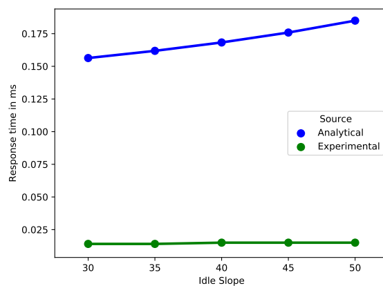
(b) Tiempo de respuesta en milisegundos de tráfico de clase B. En las cuatro transmisiones distintas se varía la pendiente de inactividad para el tráfico de clase A que fue transmitido en simultáneo.
