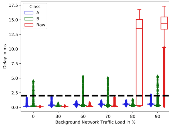
(a) Diagrama de caja para la topología Anillo. En este diagrama se presenta la demora de un extremo a otro para cada tipo de tráfico. La línea punteada negra refleja la demora máxima asegurada por AVB/TSN para tráfico de clase A.
