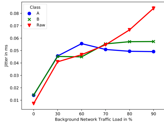
(b) Variación de jitter en milisegundos de tráfico AVB/TSN y tráfico Ethernet (Raw) para distintos porcentajes de tráfico de saturación inyectado. Los resultados fueron tomados con un intervalo de confianza de 95 %.
