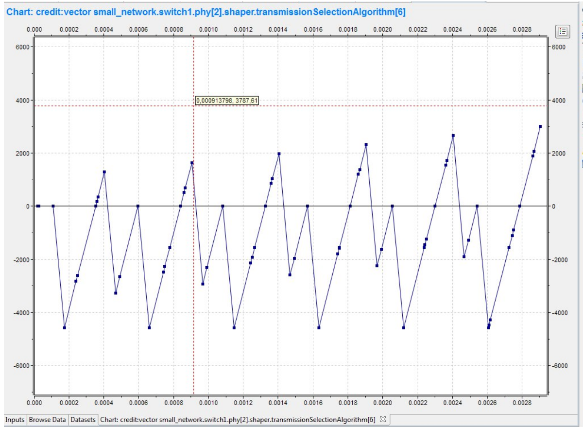
Figura 2.6: Resultado de la simulación correspondiente a la topología Estrella. Se muestra la variación en la cantidad de créditos en base al tiempo transcurrido en la clase B de tráfico transmitida en el puerto 2 del switch 1. Una transmisión dura desde el punto mínimo al punto máximo de créditos. Una vez que se transmite toda la información, la cantidad de créditos incrementa hasta alcanzar el valor 0. Cuando incrementa hasta un máximo local mayor a 0 es porque no puede transmitir, dado que el puerto está ocupado con otra tarea. Puede observarse que la cantidad máxima de créditos va aumentando con el paso del tiempo, lo que refleja un aumento en la demora en el puerto para transmitir la clase de tráfico correspondiente. Además se puede ver que la cantidad de créditos gastados por transmisión es siempre la misma, por lo que siempre se envía la misma cantidad de datos.
